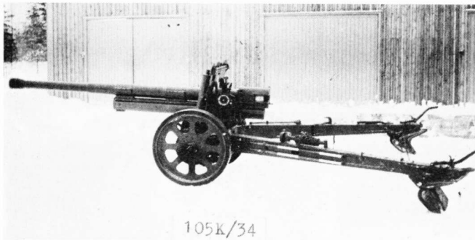
105K/34 oli valmistettu Ruotsin Boforsilla. Se painoi 4000 kg, ammuksen lähtönopeus oli 764 metriä sekunnissa ja virallinen ampumaetäisyyden maksimi 16,2 km
