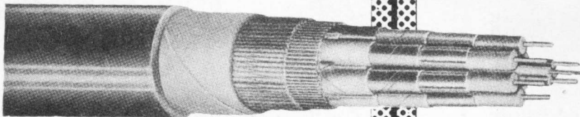
6-putkinen yhdistetty pienoiskoaksiaali- ja verkkoryhmäkaapeli
